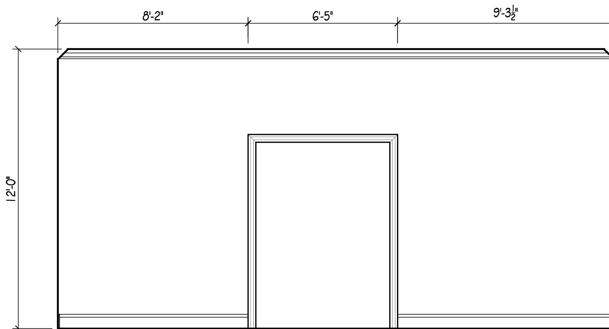
19 - DEN SCALE: 1/4" = 1'-0"
