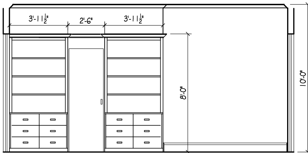
2.01 - BED2 SCALE: 1/4" = 1'-0"
