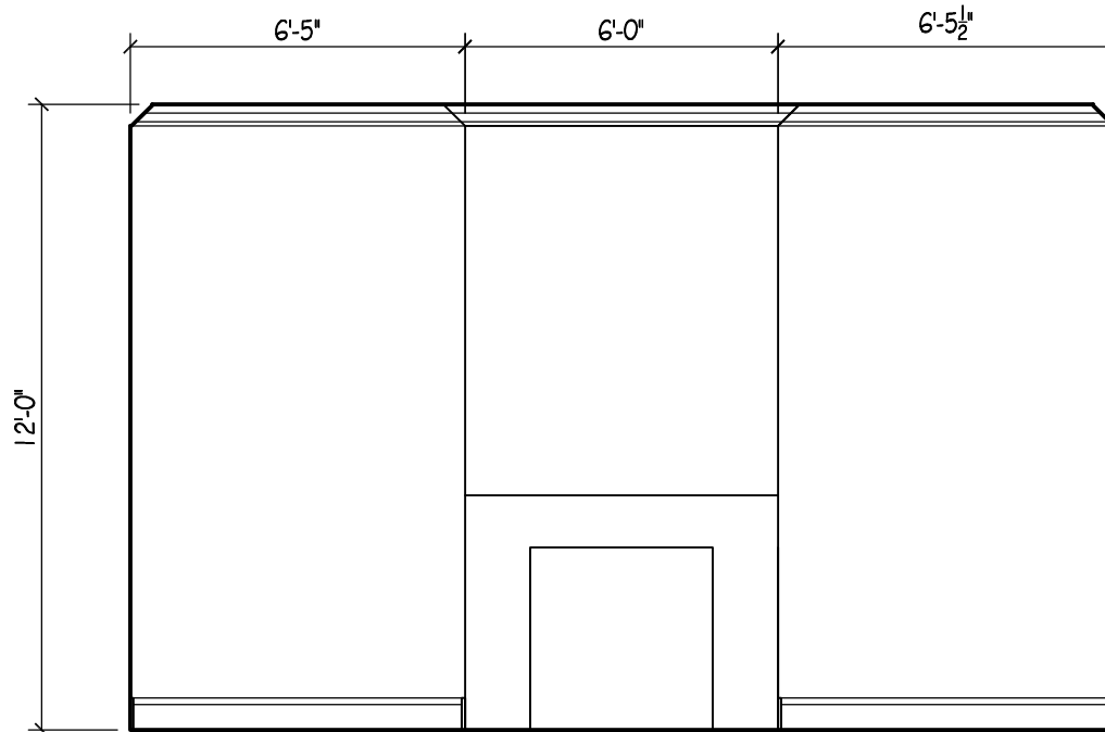
22 - DEN SCALE: 1/4" = 1'-0"
