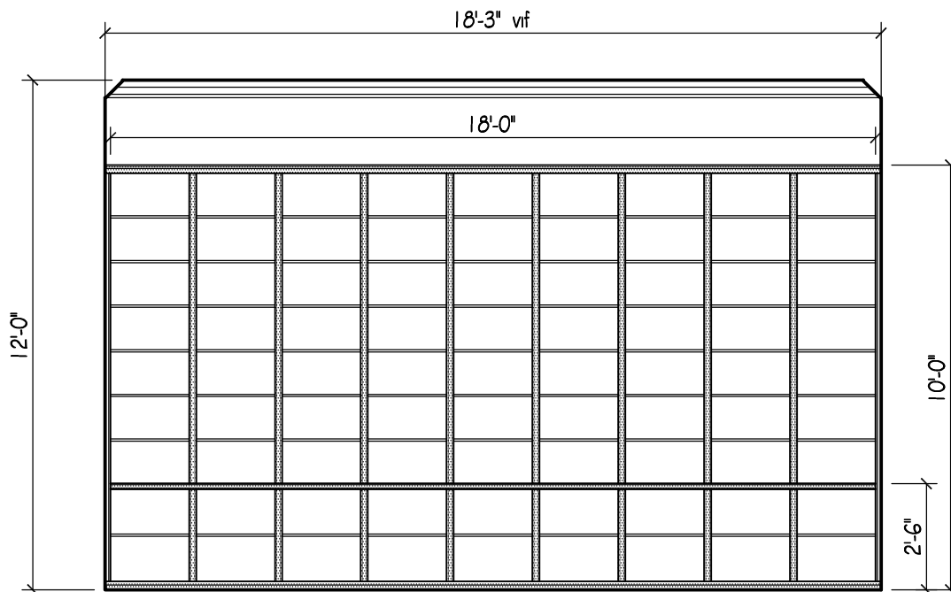
15 - DINING SCALE: 1/4" = 1'-0"
