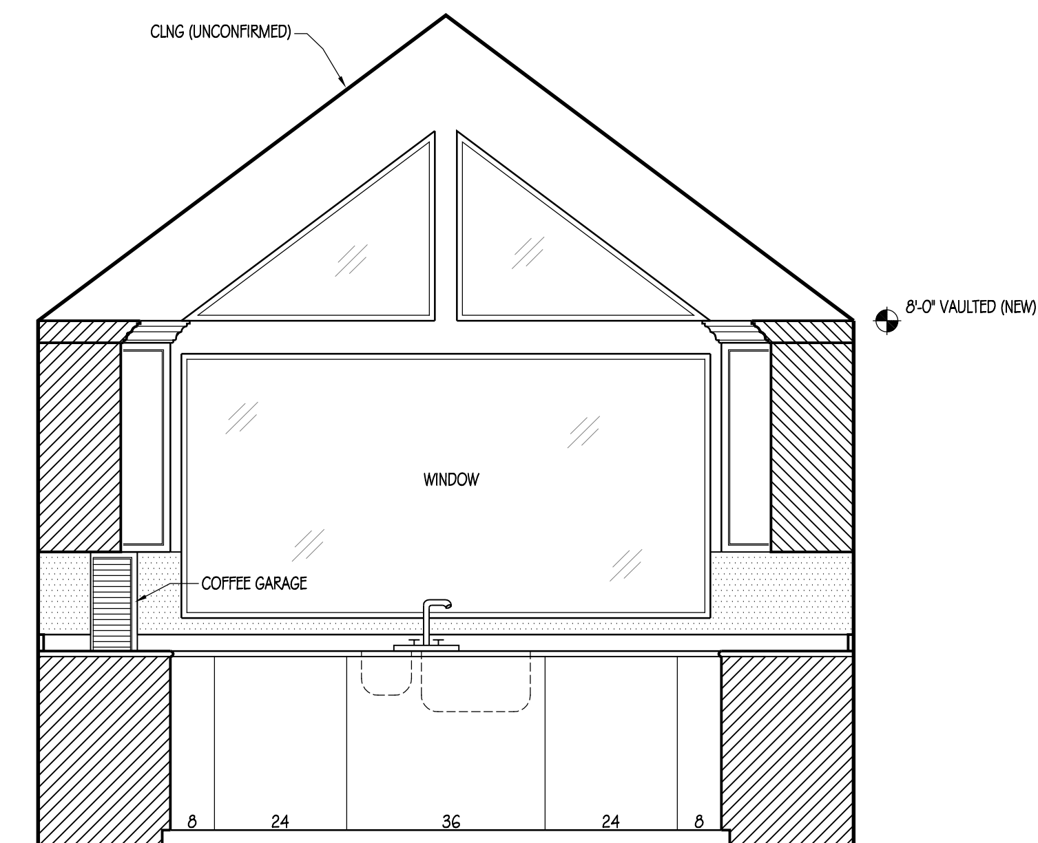
ELEVATION 03 SCALE: 1/2"
